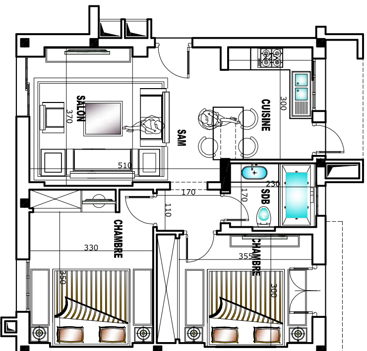
Plan aménagement Appart SC2 RDC
